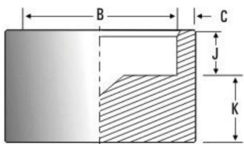
SOCKET WELD ДАНЦЕ P
