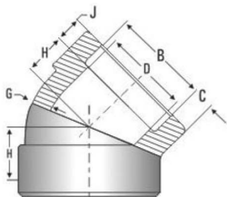
SOCKET WELD КОЛЕНО 45° SOCKET WELD ELBOW 45°
