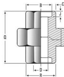
SOCKET WELD ХОЛЕНДЕР SOCKET WELD UNION
