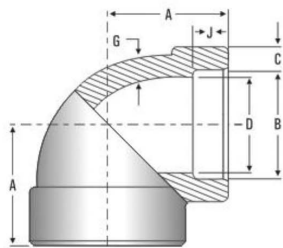
SOCKET WELD КОЛЕНО 90° SOCKET WELD ELBOW 90°
