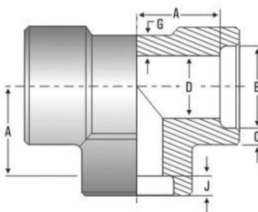
SOCKET WELD T ШТИК SOCKET WELD TEE
